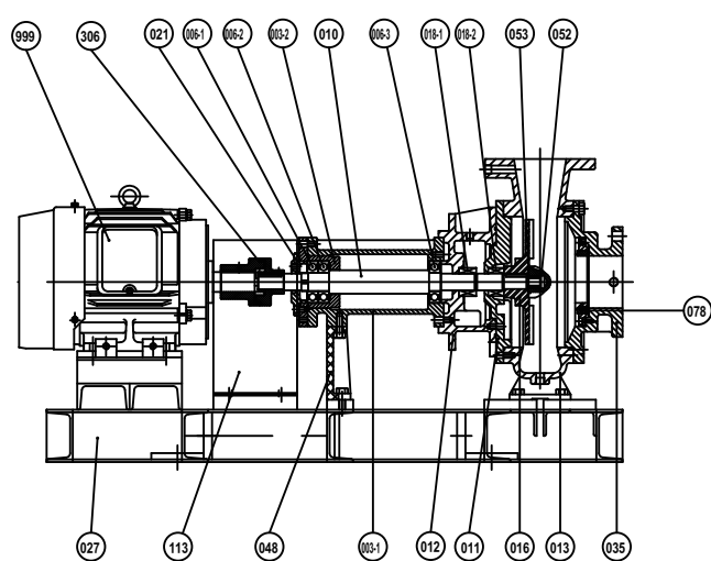
CHD(SS)乾井臥式聯軸不堵塞污物(泥)泵
