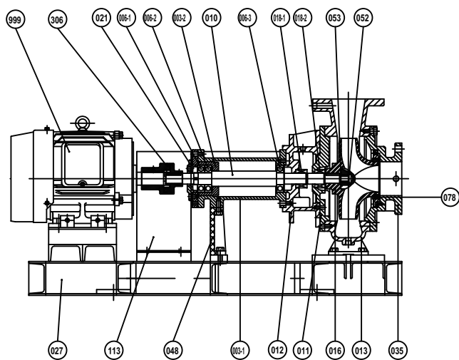
CHD乾井臥式聯軸不堵塞污物(泥)泵
