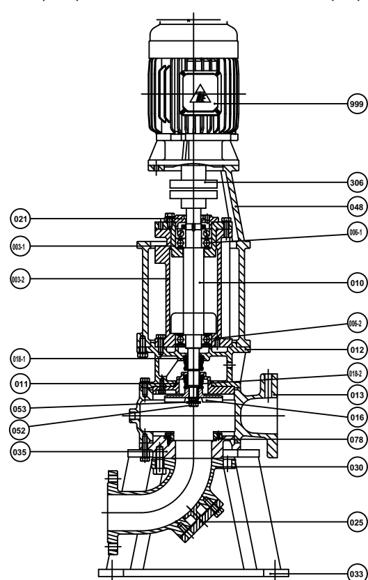
CVD(SS)乾井立式聯軸不堵塞污物(泥)泵
