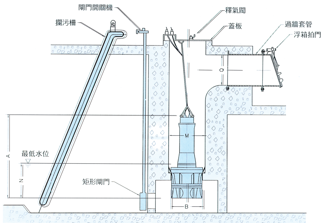
圖一：RC製井桶式施工大樣圖
