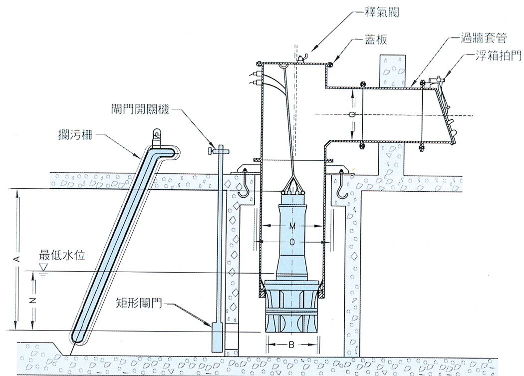
圖二：鋼製井桶式施工大樣圖
